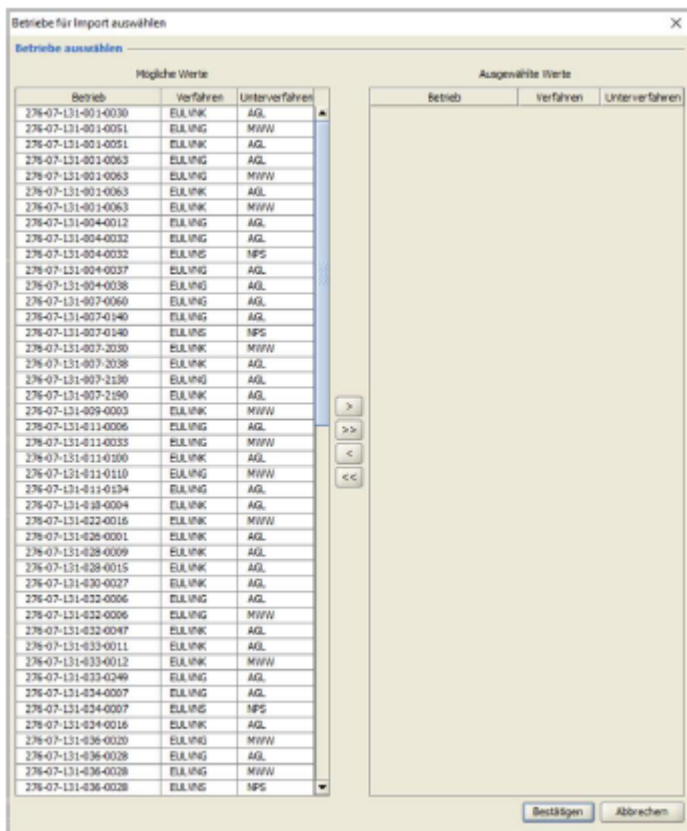
Abbildung 4: LBD-Dialogfenster Betriebsauswahl
