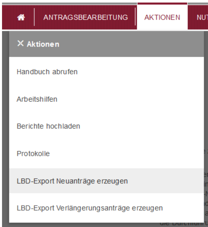
Abbildung 1: LBD-Export erzeugen
