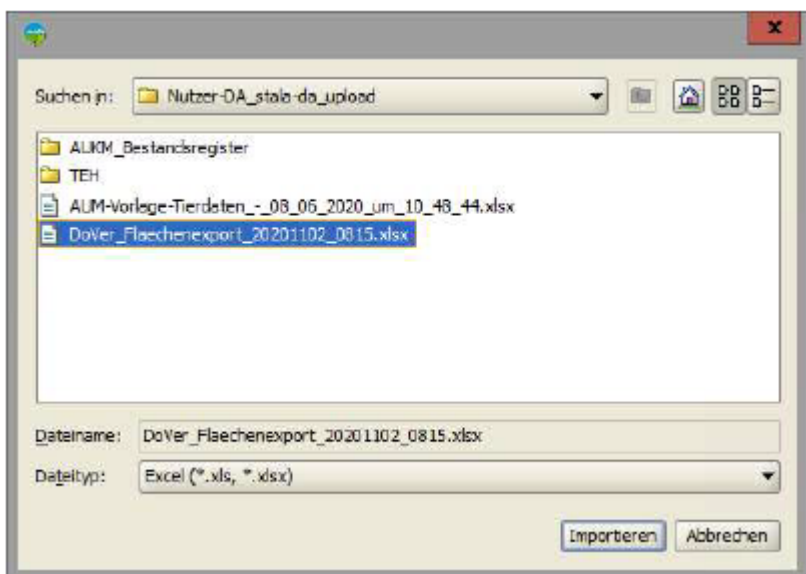
Abbildung 3: LBD-Importfenster Dateiauswahl
