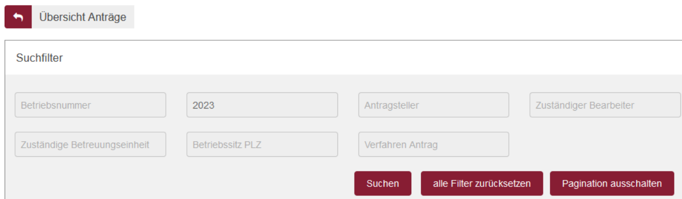
Abbildung 1: Suchfilter Anträge
